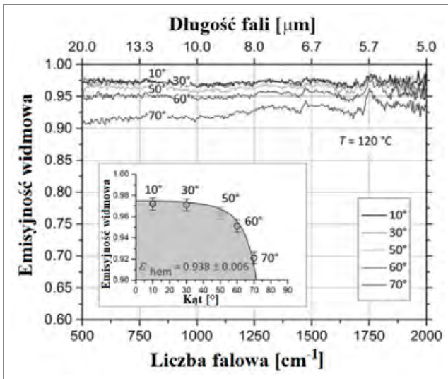
Rys. 4. Emisyjność farby Nextel 811-21 w funkcji kąta [1] Fig. 4. Nextel 811-21 paint emissivity as an angle function [1]
