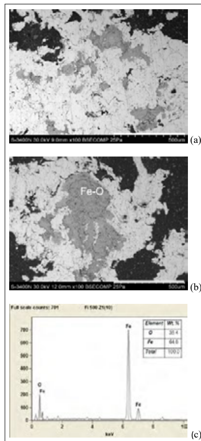
Fig. 6. Microstructure observed on flat spot-sections using the SEM microscope: a, b) two different "spots" of the sample DN500; c) EDS analysis of the ferric oxide area (magnification bar of 0.5 mm) Ryc. 6. Mikrostruktura zaobserwowana na płaskich przekrojach plamkowych za pomocą mikroskopu SEM: a, b) dwa różne „punkty” próbki DN500; c) Analiza EDS obszaru tlenku żelaza (pasek powiększenia 0,5 mm)
