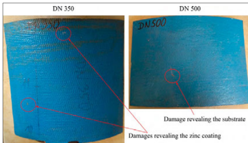
Fig. 2. Images of the material cut from the pipes with diameter of 350 mm and 500 mm Ryc. 2. Zdjęcia materiału wyciętego z rur o średnicy 350 mm i 500 mm
