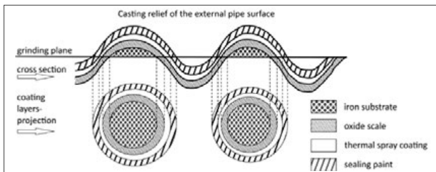
Fig. 4. Diagram of the grinding plane tangential to the external pipe surface - theoretical appearance of flat "spots" for a further metallographic study has been shown. Ryc. 4. Schemat płaszczyzny szlifowania stycznej do powierzchni zewnętrznej rury - pokazano teoretyczny wygląd płaskich „plam” do dalszych badań metalograficznych.
