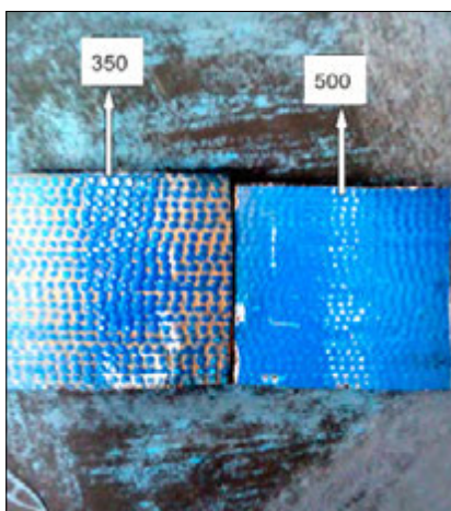
Fig. 3. Images of samples abrasion using paper of 1000#. Blue sediment for the pipe DN 350 and gray sediment for DN 500, respectively. Ryc. 3. Widok próbek ścieranych na papierze o gradacji 1000#. Niebieski osad dla rury DN 350 i szary osad odpowiednio dla rury DN 500.
