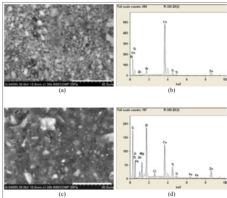
Fig. 8. Paints morphology and a chemical composition: a) the sample DN 350, b) the respective EDS analysis, c) the sample DN500, d) the respective EDS analysis (magnification scale of 30 mm) Ryc. 8. Morfologia farb i skład chemiczny: a) próbka DN 350, b) odpowiednia analiza EDS, c) próbka DN500, d) odpowiednia analiza EDS (skala powiększenia 30 mm)
