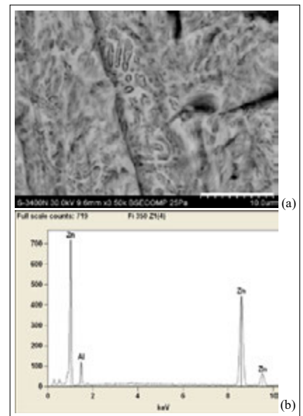
Fig. 7. Microstructure of the Zn-Al coating: a) flat section of the sample DN500 (magnification scale of 10 mm), b) EDS analysis of the coating Ryc. 7. Mikrostruktura powłoki Zn-Al: a) płaski przekrój próbki DN500 (skala powiększenia 10 mm), b) Analiza powłoki EDS
